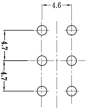
P.C.B LAYOUT BOTTOM VIEW 注“*”表示关键尺寸 (6个)
