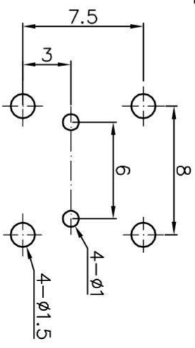
PCB线路板安装图(±0.1)
