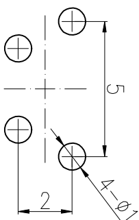
PCB线路板安装图(±0.1)
