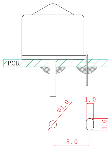
PCB焊锡插脚孔位
