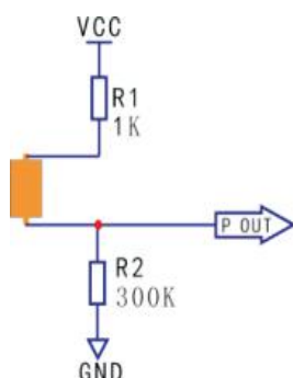
开关测试图
