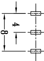
P.C.B LAYOUT
