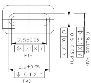
DETAIL: B-B SCALE: 2:1
