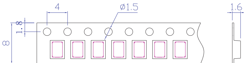
编带示意图
