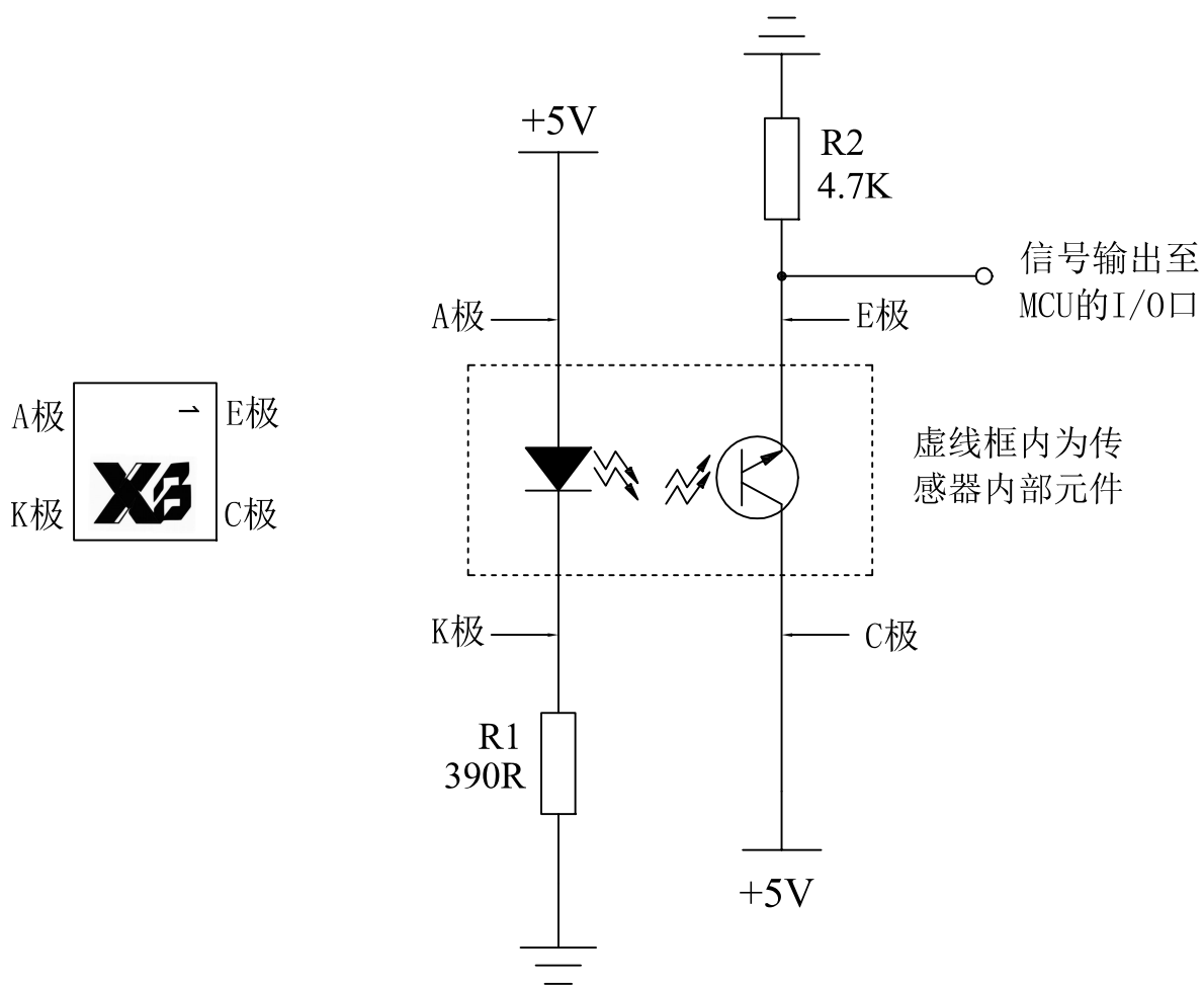
传感器内部电路元件与外部引脚连接图 R1与R2为外接电阻
