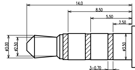
( \phi 3.5\text{mm} 4 POLE PLUG DETAIL DRAWING)
