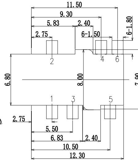
P.C.B LAYOUT TOP VIEW 正贴
