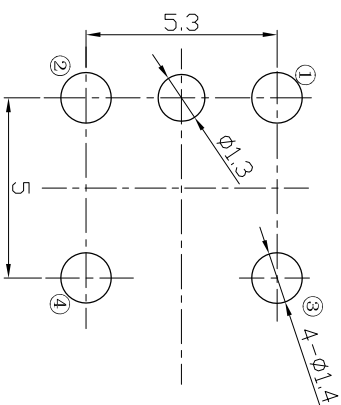
安装位置图
