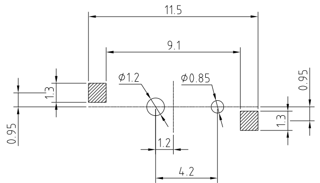
印制电路板及焊接安装孔参考图 （自A方向看）
