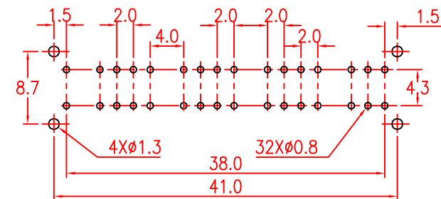
P.C.B LAYOUT
