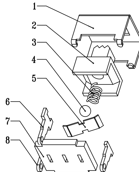
产品结构示意图
