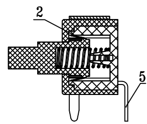
截面 A-A
