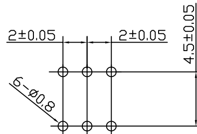
P.C.B 设计参考尺寸
