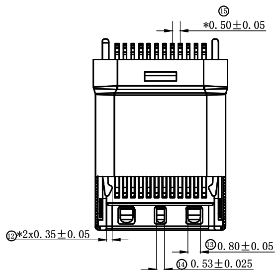
截面 E-E
