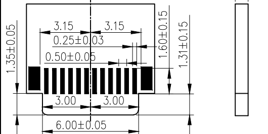
PCB板的外形
