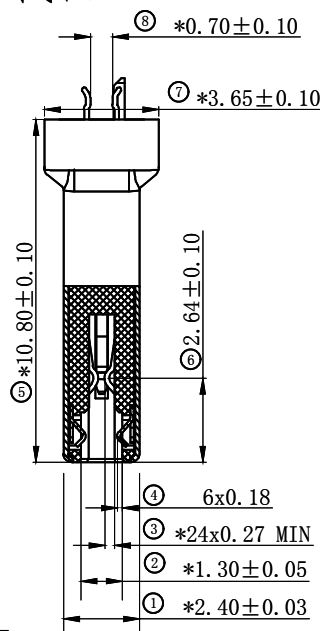
截面 A-A
