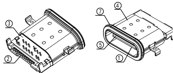
3D 示意图(组装后带防水圈)
