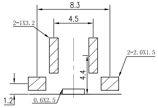
PCB线路板安装图(±0.1)
