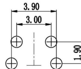
PCB线路板安装图(±0.1)
