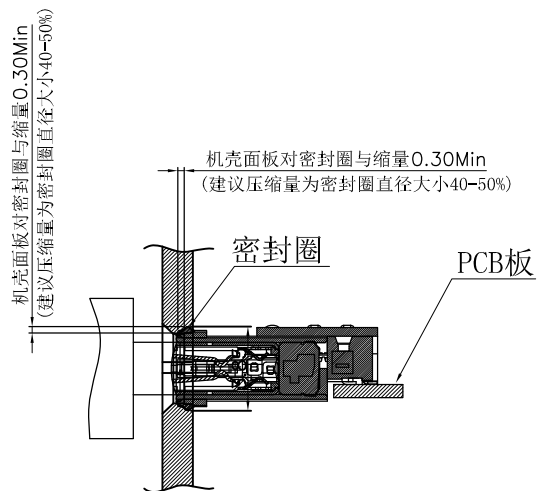
组装面板后公母头对插示意图
