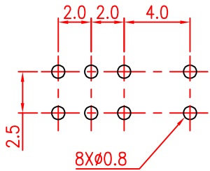
P.C.B LAYOUT
