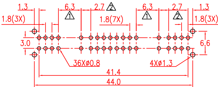
P.C.B. LAYOUT
