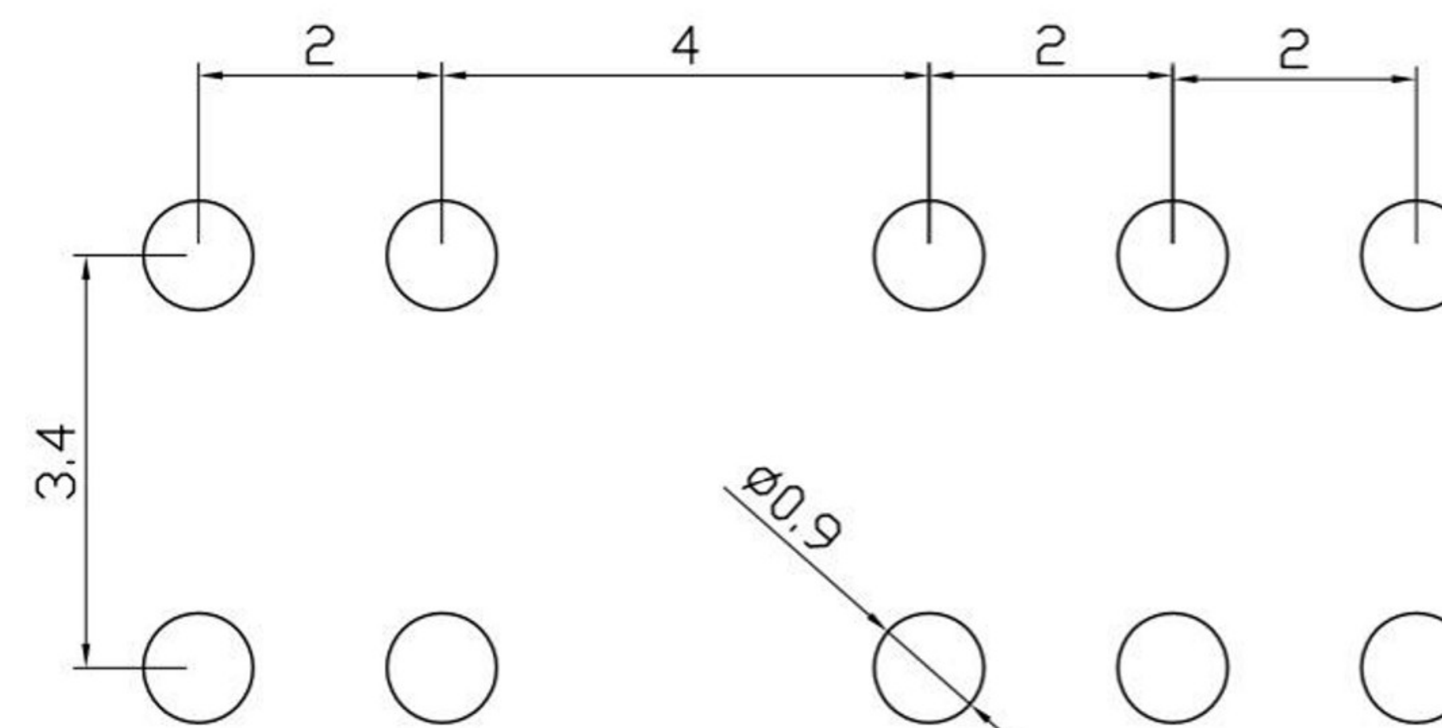
安装图 (PCB LAYOUT PLAN)
