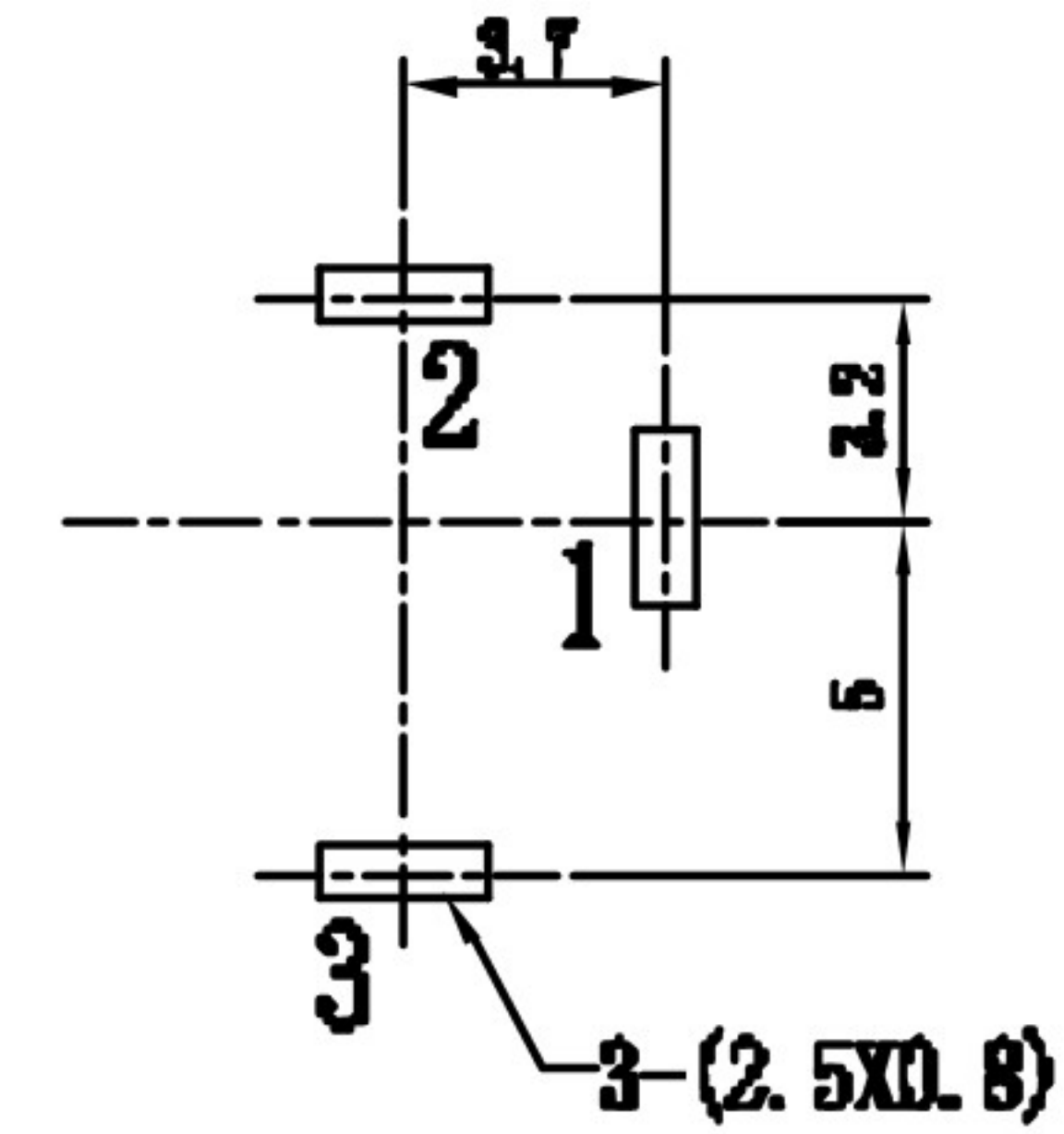
线路板开孔尺寸 P.C.B LAYOUT
