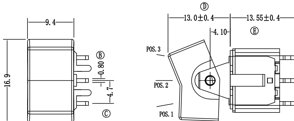
标注: ①-⑩为重点检测尺寸
