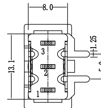
A-A剖面
