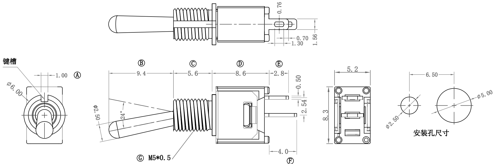
手柄位置及导通端子示意图
