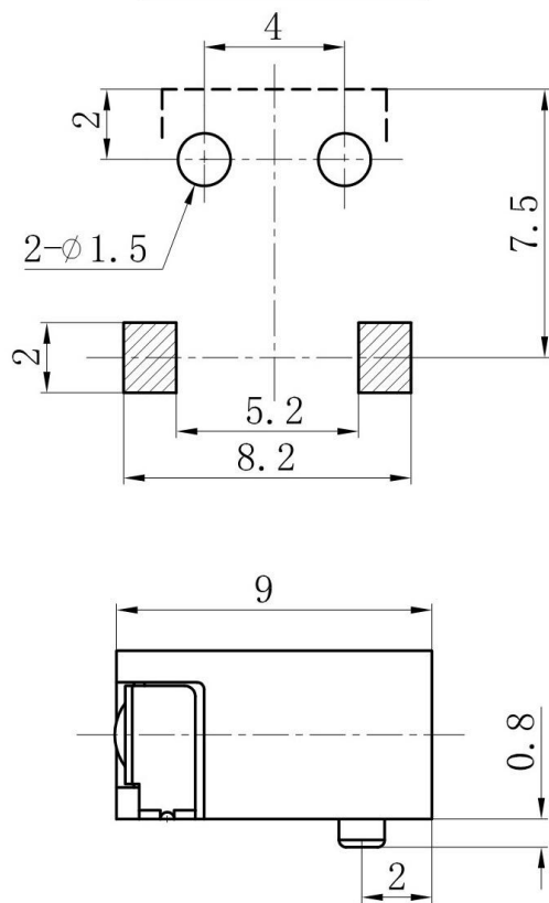
PCB板位置尺寸
