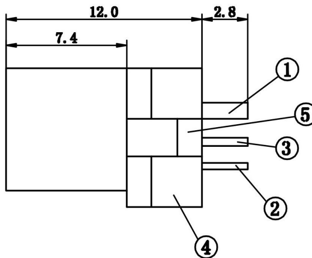
电路结构示意图
