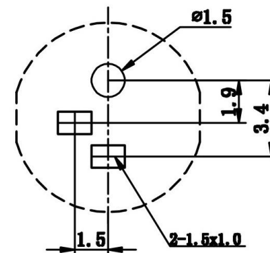
线路板安装尺寸示意图
