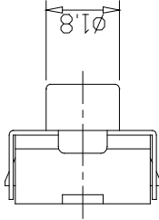
P.C.B LAND DIMENSION
