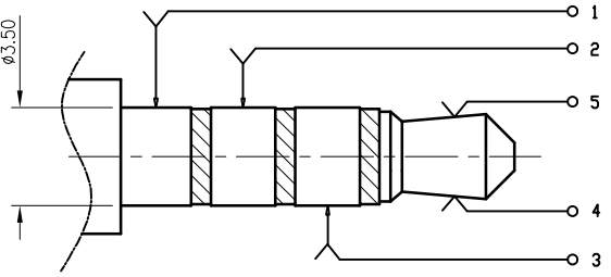
PULG SCHEMATIC
