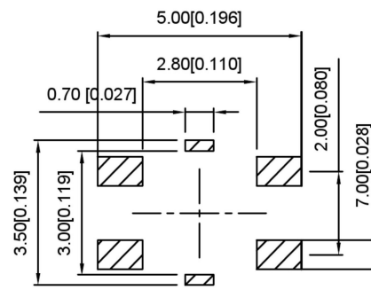
PCB 焊接图
