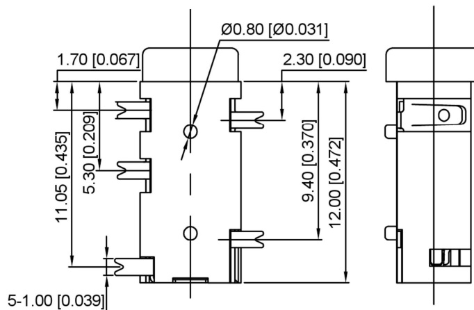
五金帽截面图
