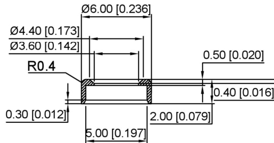
五金帽截面图
