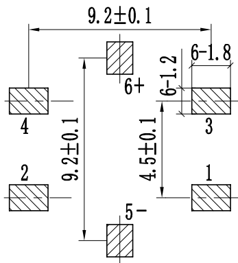
元件面孔位图
