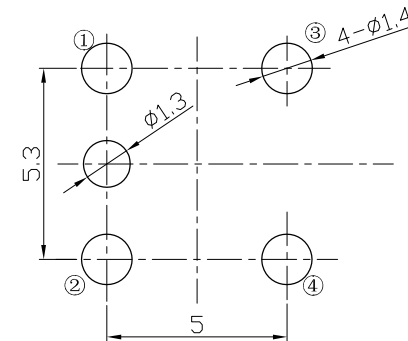
安装位置图
