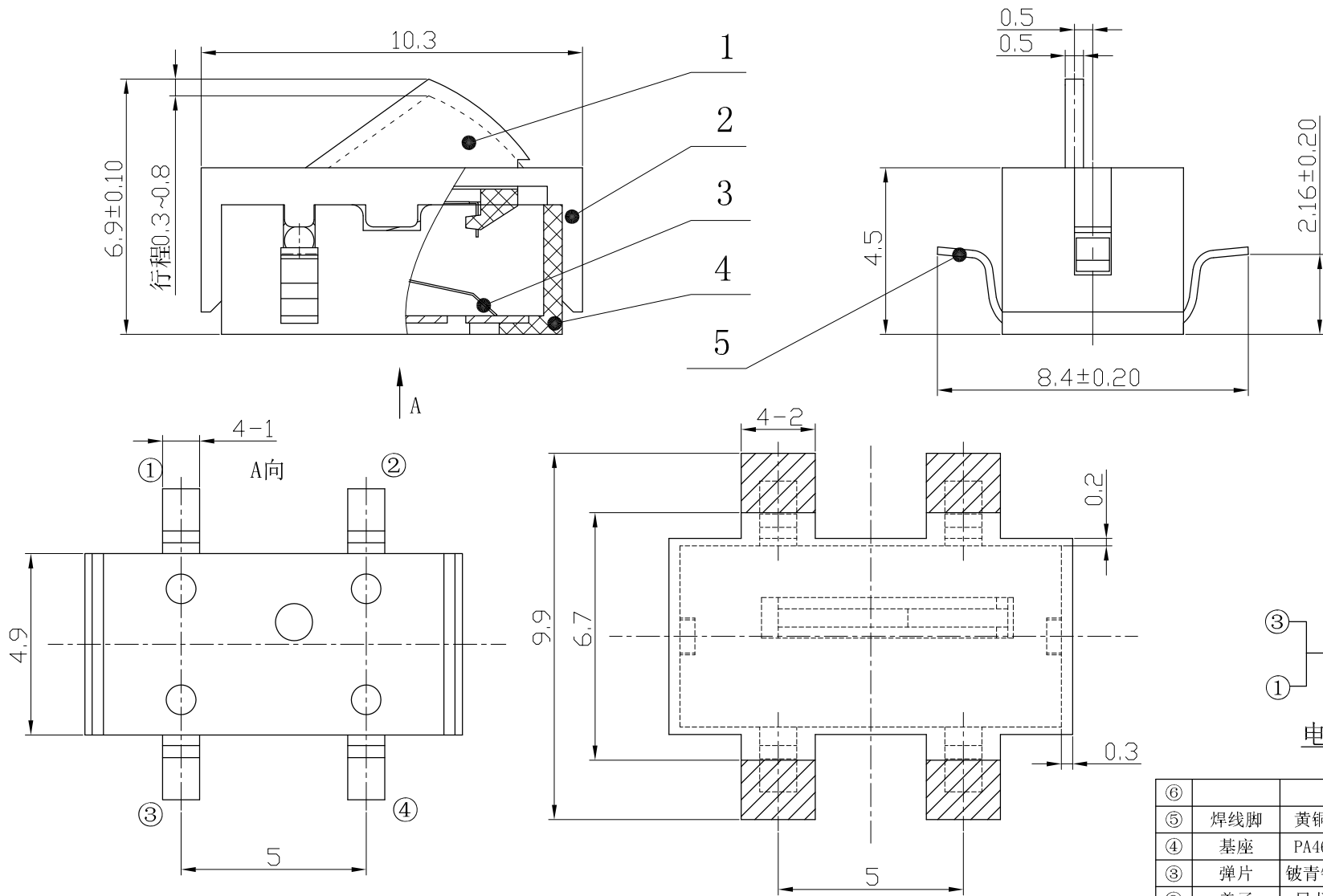
安装尺寸图
