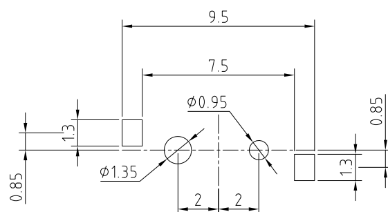
印制电路板及焊接安装孔参考图 (自A方向看)
