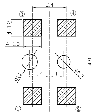
安装位置图
