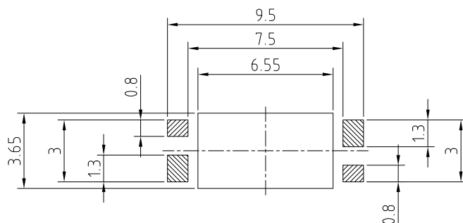
印制电路板及焊接安装孔参考图 (自A方向看)
