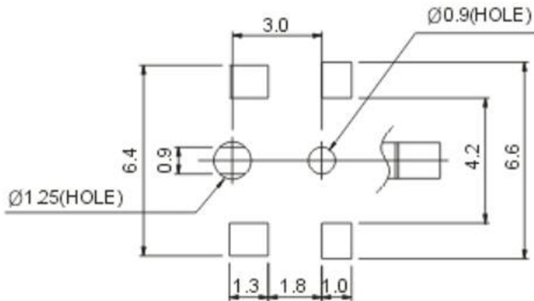
P.C.B LAND DIMENSION
