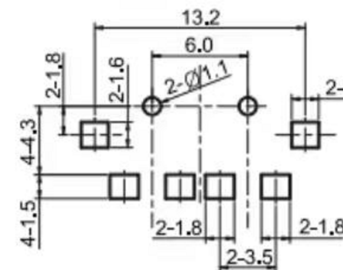
P.C.B LAND DIMENSION
