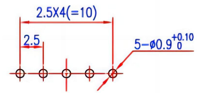
安装尺寸图
