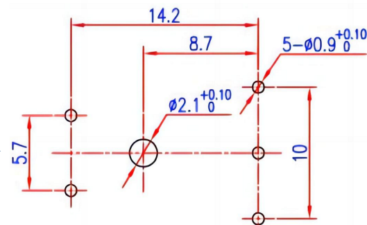
安装尺寸图
