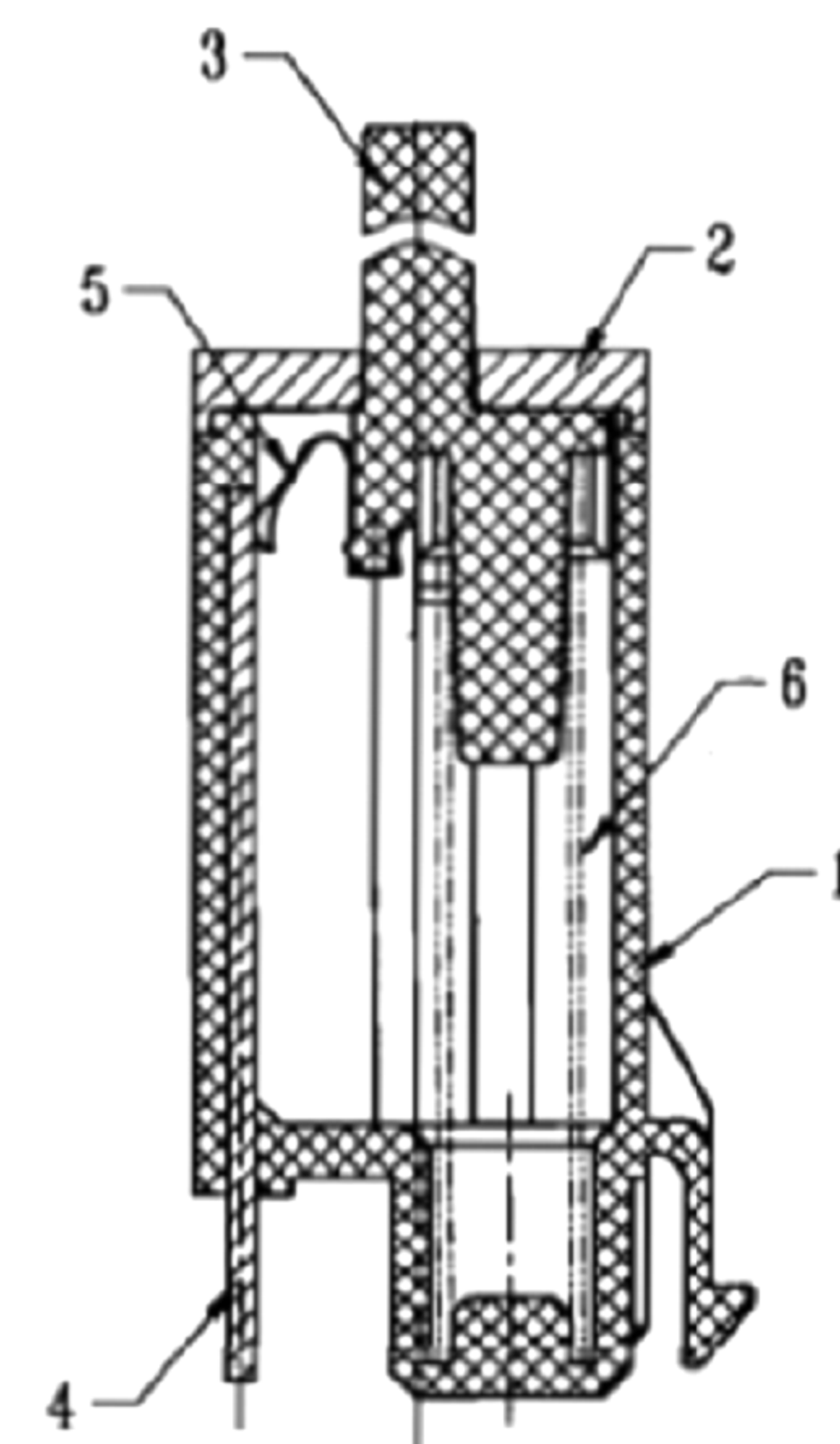
內部構造圖
