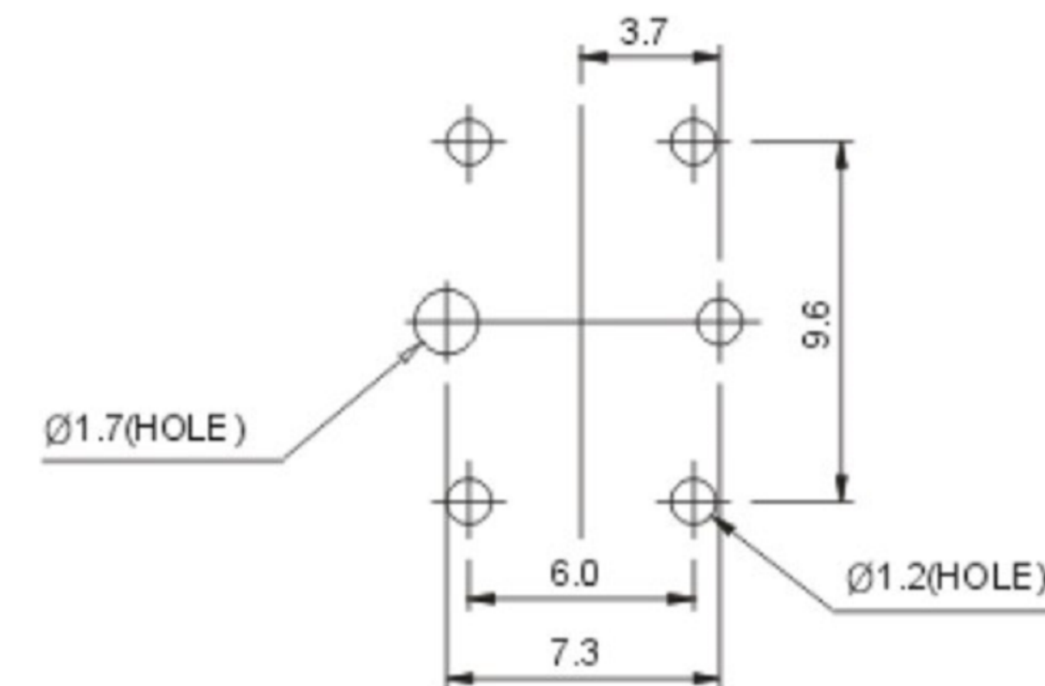
P.C.B HOLE DIMENSION
