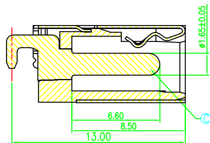
SECTION A-A 8.80
