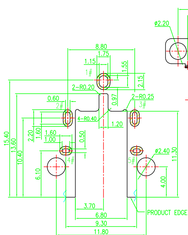
SECTION A-A
