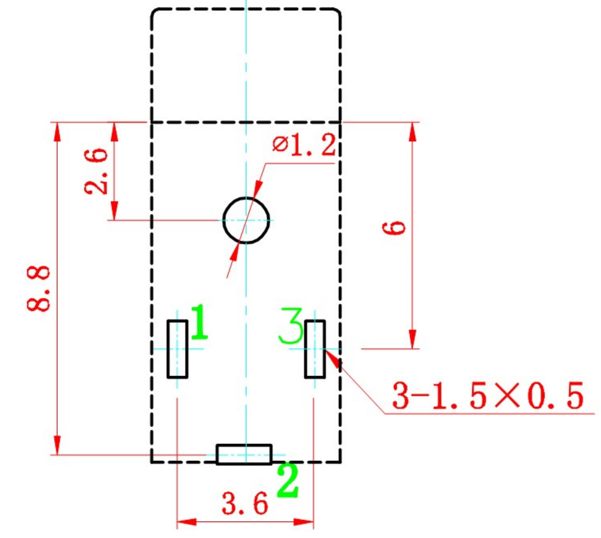
线路板开孔尺寸 (TOP VIEW)
