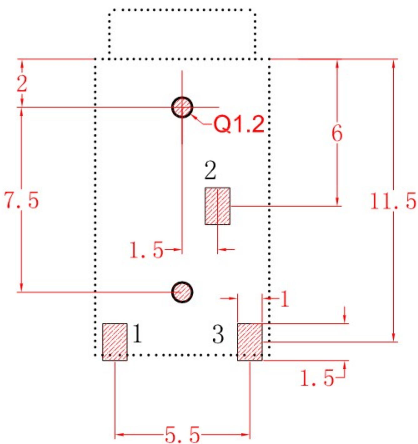
线路板开孔尺寸
